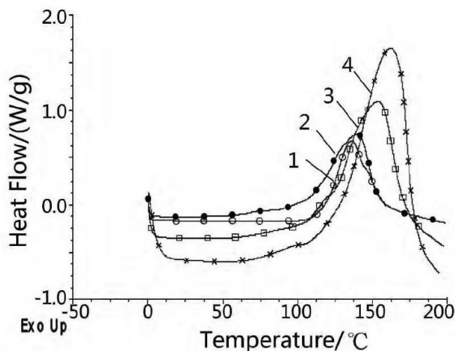
图表27：18-冠醚-6 对氰基丙烯酸酯胶固化反应动力学的影响
