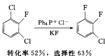
图表16：季鎔盐催化 Hallex 反应式
