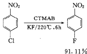
图表17：季铵盐催化 Hallex 反应式
