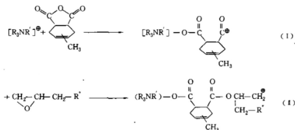
图表25：季铵盐对环氧树脂固化反应体系促进机理
