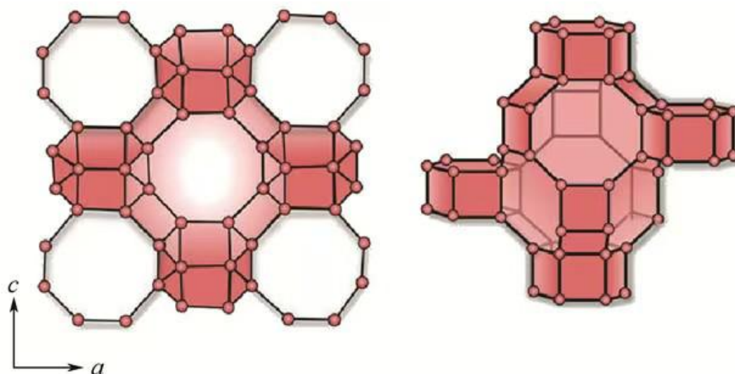
图表23：SSZ-13 分子筛结构
