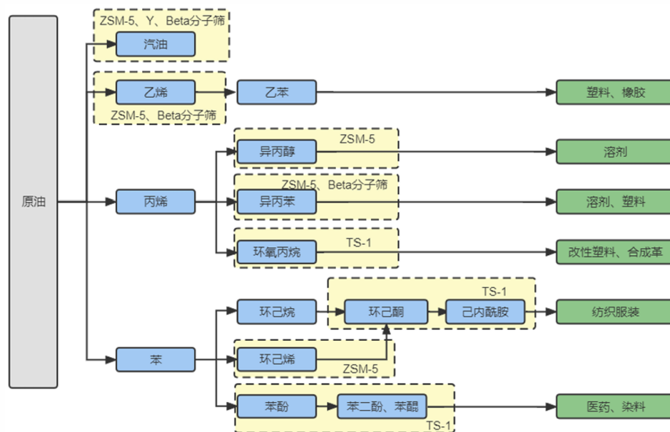
图表21：TS-1、ZSM-5、Beta 分子筛石油化工领域主要应用方向
