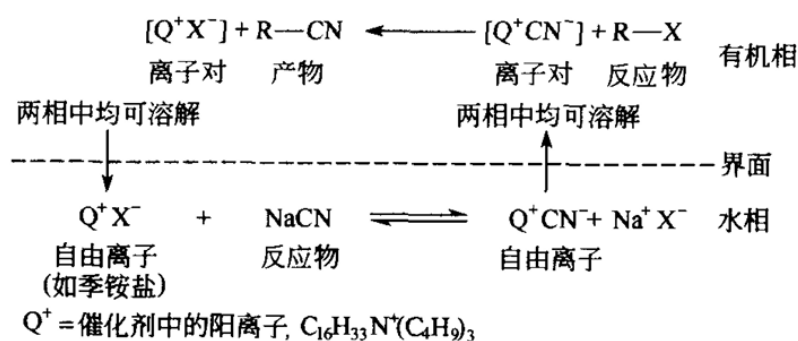
图表14：相转移催化及作用机理（以季铵盐为例）
