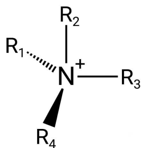
图表33：四丁基铵阳离子结构图（R 1 至R 4 为正丁基）
